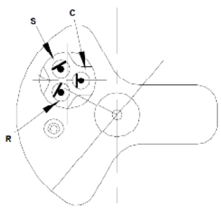
Anschlussbild Verdichter
